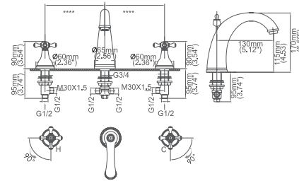
Model No:C-16 Lavatory Faucet
