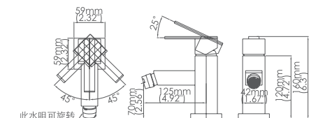
Model No:H-40-HC Bidet Faucet
