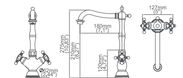
Model No:C-34 Lavatory Faucet
